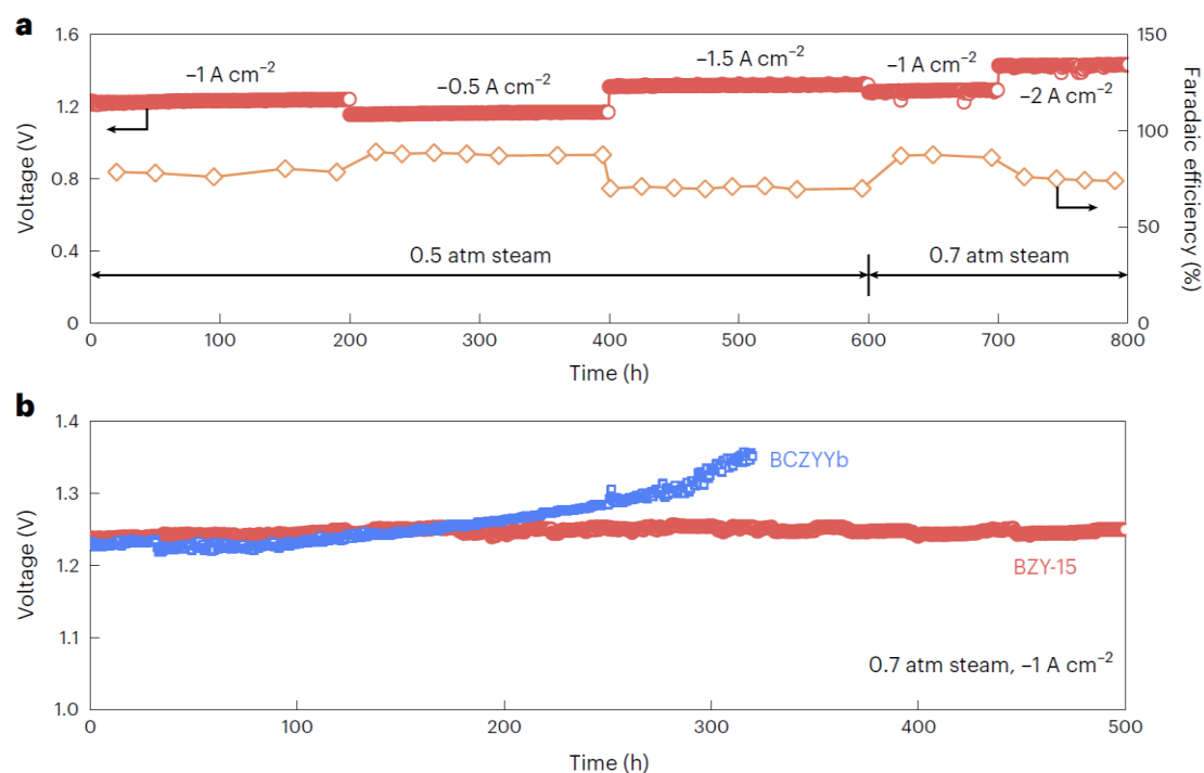
图 2. 锆酸钡基陶瓷质子膜电池具有优异的电解稳定性
