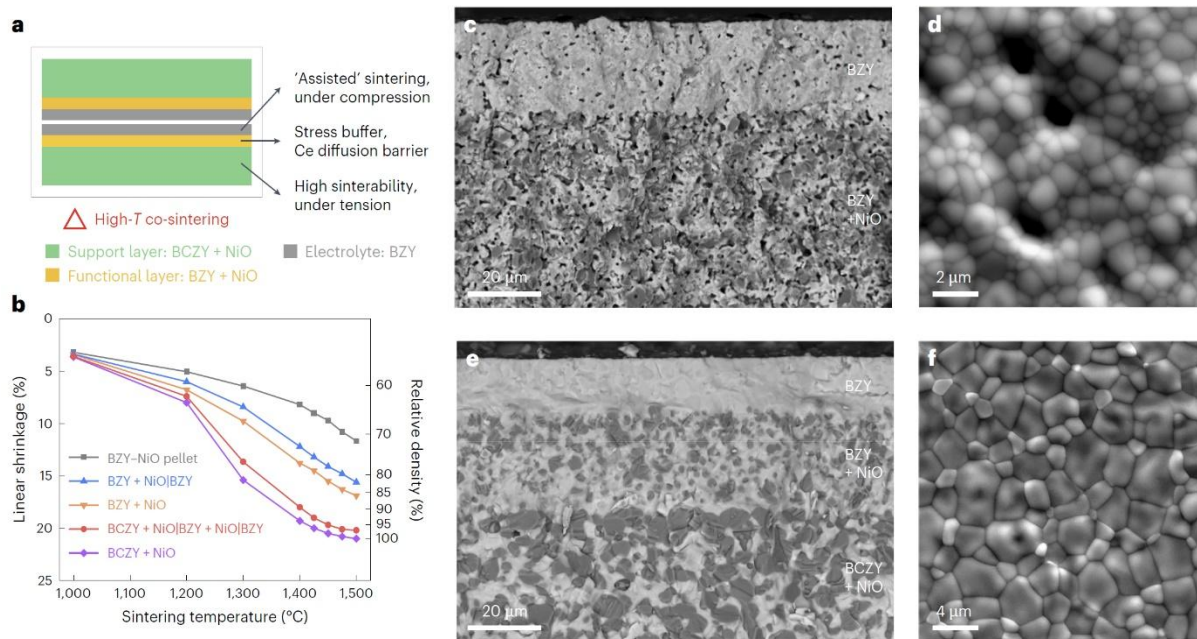
图 1. 锆酸钡基陶瓷质子膜多层共烧技术
